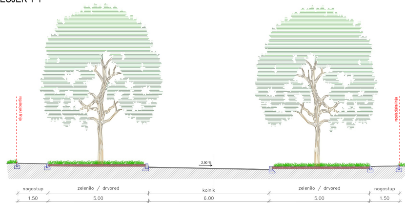
NORMALNI PRESJEK 2-2
