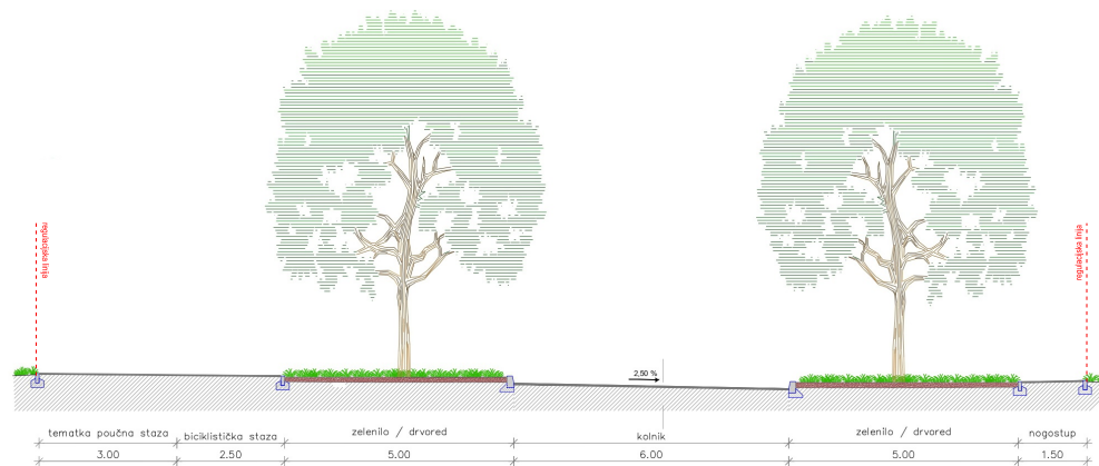
NORMALNI PRESJEK 3-3
