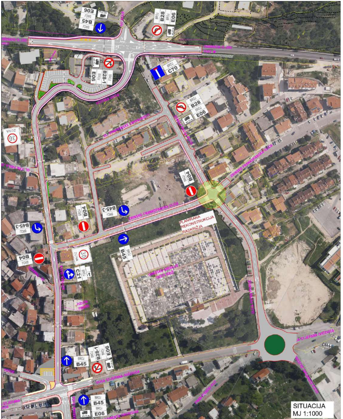
Spoj Kotiške ulice na magistralu_Varijanta 4_20.01.2024_projektant R.Gusić, dipl.ing.građ. "Platea" d.o.o. Split
